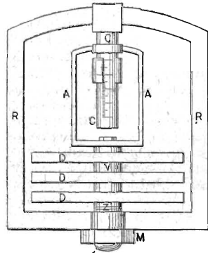
Фиг. 4. Лотъ Голфгартнера.
