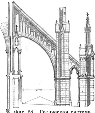
Фиг. 28. Готическая система коштфорсовъ.
