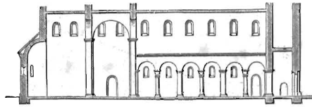
Фиг. 18. Продольный разрез романской базилики.
