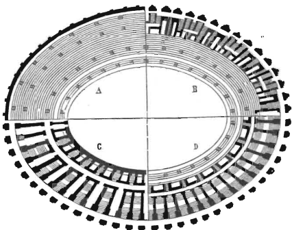
Рис. 2. Планъ амфитеатра въ Нимѣ. А на высотѣ послѣднихъ ступеней наружнаго круга, В на высотѣ второго, С на высотѣ первого круга, D разрѣзъ на уровнѣ земли.
