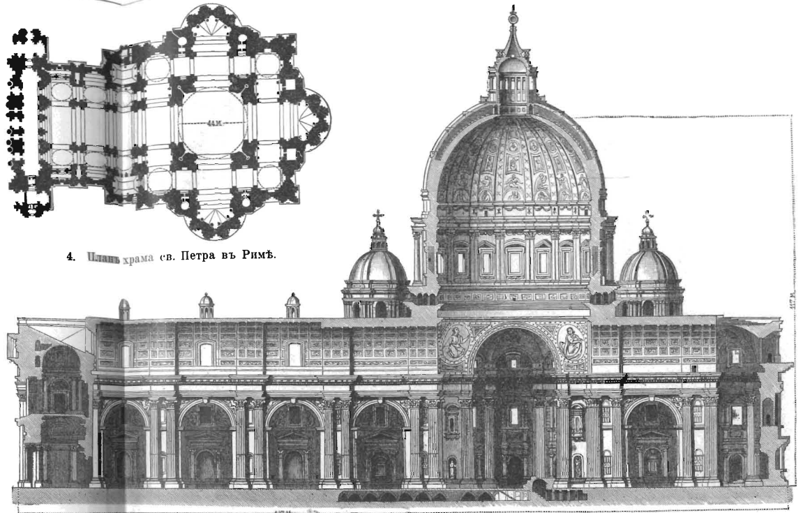
Рис. 3. Храмъ св. Петра въ Римѣ. Продольный разрѣзъ. Къ рис. 2—4. Начатъ Браманте въ 1506 г., продолжали: Рафаэль, Перуцци, Сангалло и въ 1546 г. Микеланджело; окончить въ 1626 г. Мадерна.
