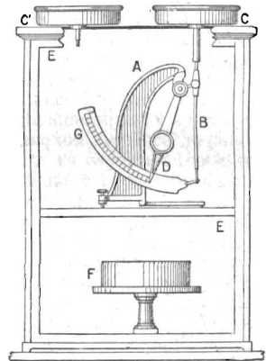
Атмометръ Вильда.
