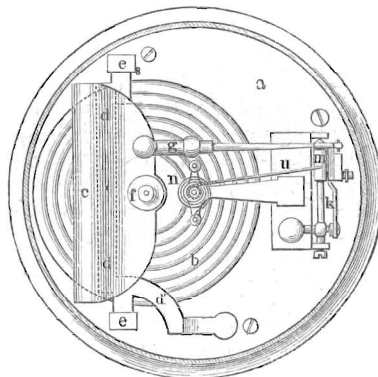
Фиг. 6. Продольный разрѣзъ. Пружинный барометръ Ноде.
