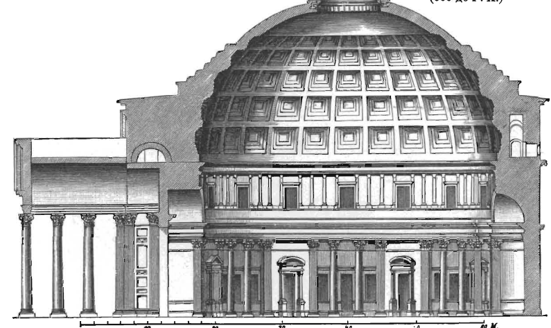
Рис. 16. Разрѣзь Пантеона въ Римѣ.
