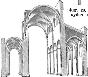
Фиг. 23. Романская система кресто-рых сводовъ.
