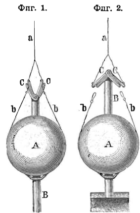
Лотъ Брука.
