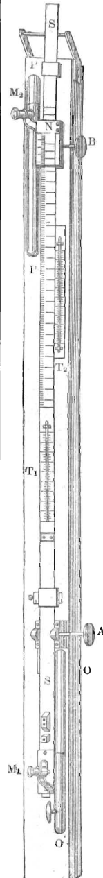
Сифонный барометръ.
