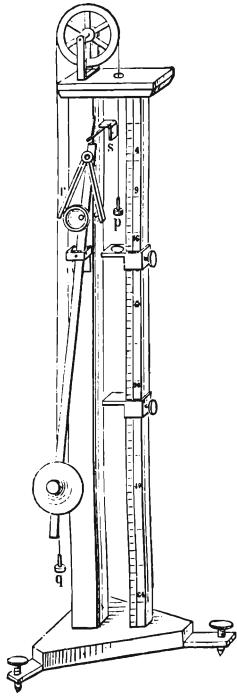
Машина Atwood'a для измѣр. силы паденія.
