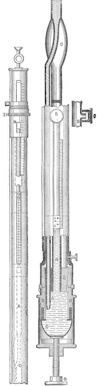
Сифонный барометръ съ чашечкой.
