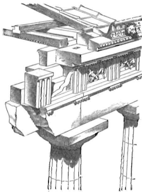
Фиг. 5. Дорическая крыша и балки.
