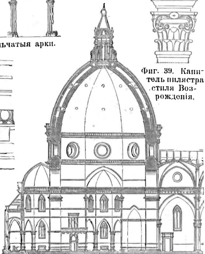
Фиг. 40. Разрезъ Флорентійскаго собора.
