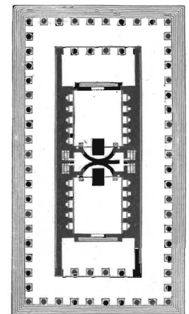
Рис. 18. Планъ храма Венеры и Ромы.
