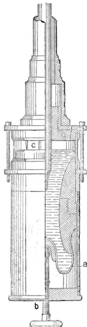
Фиг. 1 и 2. Переносный барометръ Фортина.
