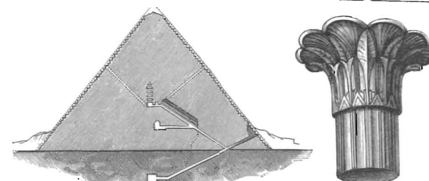
Рис. 2. Разрѣзъ большой пирамиды (Хеопса).
