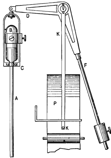
Фиг. 7. Вѣсовой барометръ.
