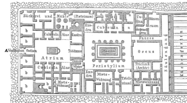
Рис. 4. Домъ Пансы въ Помпѣй. Планъ къ рис. 5 и 6.
