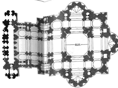
4. Планъ храма св. Петра въ Римѣ.
