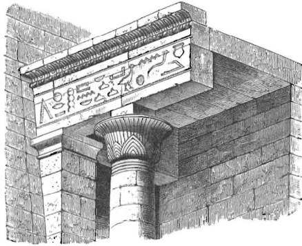
Фиг. 2. Египетские балки со столбами (пилоны) Фиг. 4. Ионич. покрытие и колоннами.
