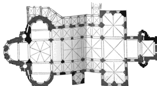
Рис. 6. Планъ церкви св. Апостоловъ въ Кельнѣ.
