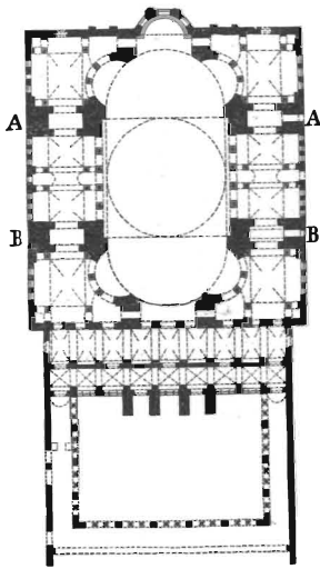
Рис. 9. Планъ собора св. Софій.
