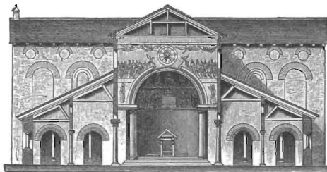
Рис. 3. Поперечное сѣченіе базилики св. Павла.
