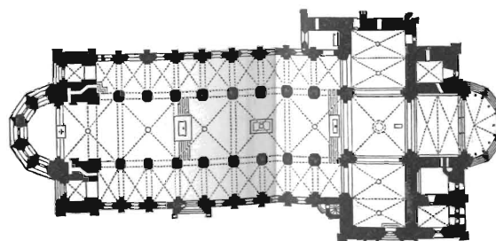
Рис. 4. Планъ Вамбергскаго собора.
