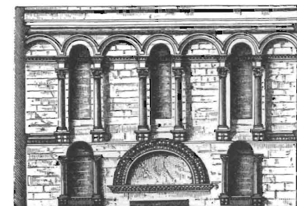
Рис. 12. Porta augusta дворца Діоклещана. Арочный карнизъ и колоннада.
