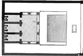
Рис. 7. Планъ этрускаго храма.
