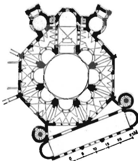
Фиг. 7. Византійск. центральнo-купольная система.
