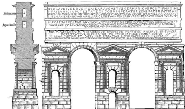
Рис. 3. Акведукъ Клавдія въ Римѣ. 52 г. по Р. X.
