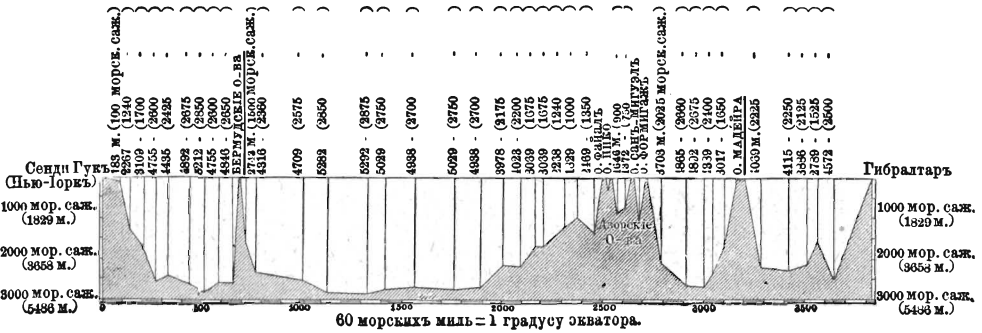
Фиг. 1. Разрѣзъ сѣв. части Атлантическаго океана черезъ Мадейру, Азорскіе и Бермудскіе о-ва до Нью-Йорка. Длина къ глубинѣ, какъ 1308:1.
