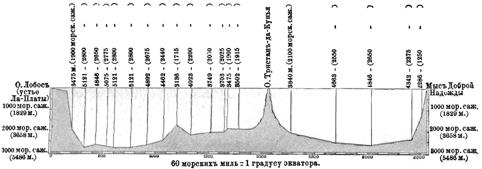
Фиг. 2. Разрѣзъ южн. части Атлантическаго океана отъ устья Ла-Платы черезъ Тристанъ-да-Кунья до мыса Доброй Надежды. Длина къ глубинѣ, какъ 1200:1.
