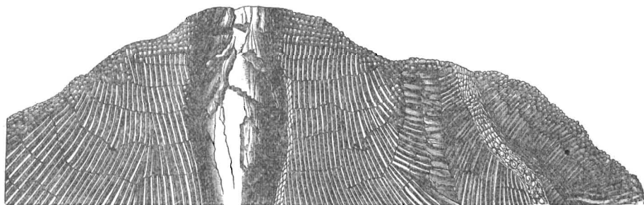
Столбчатая отдѣльность базальта у Ремагена на Рейнѣ.
