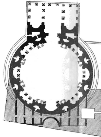
Рис. 14. Планъ Пантеона въ Римѣ.
